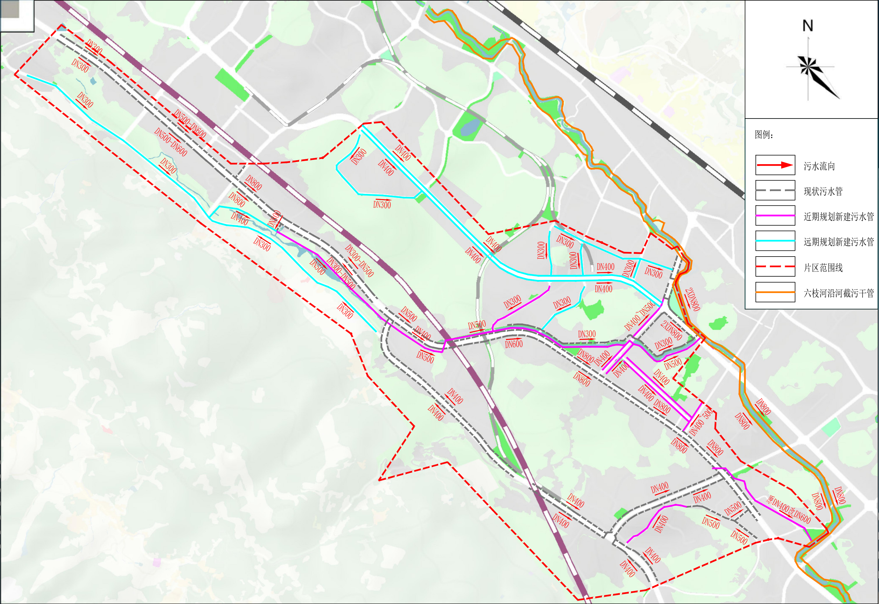
污-07 牂牁大道西片区污水管网规划图
