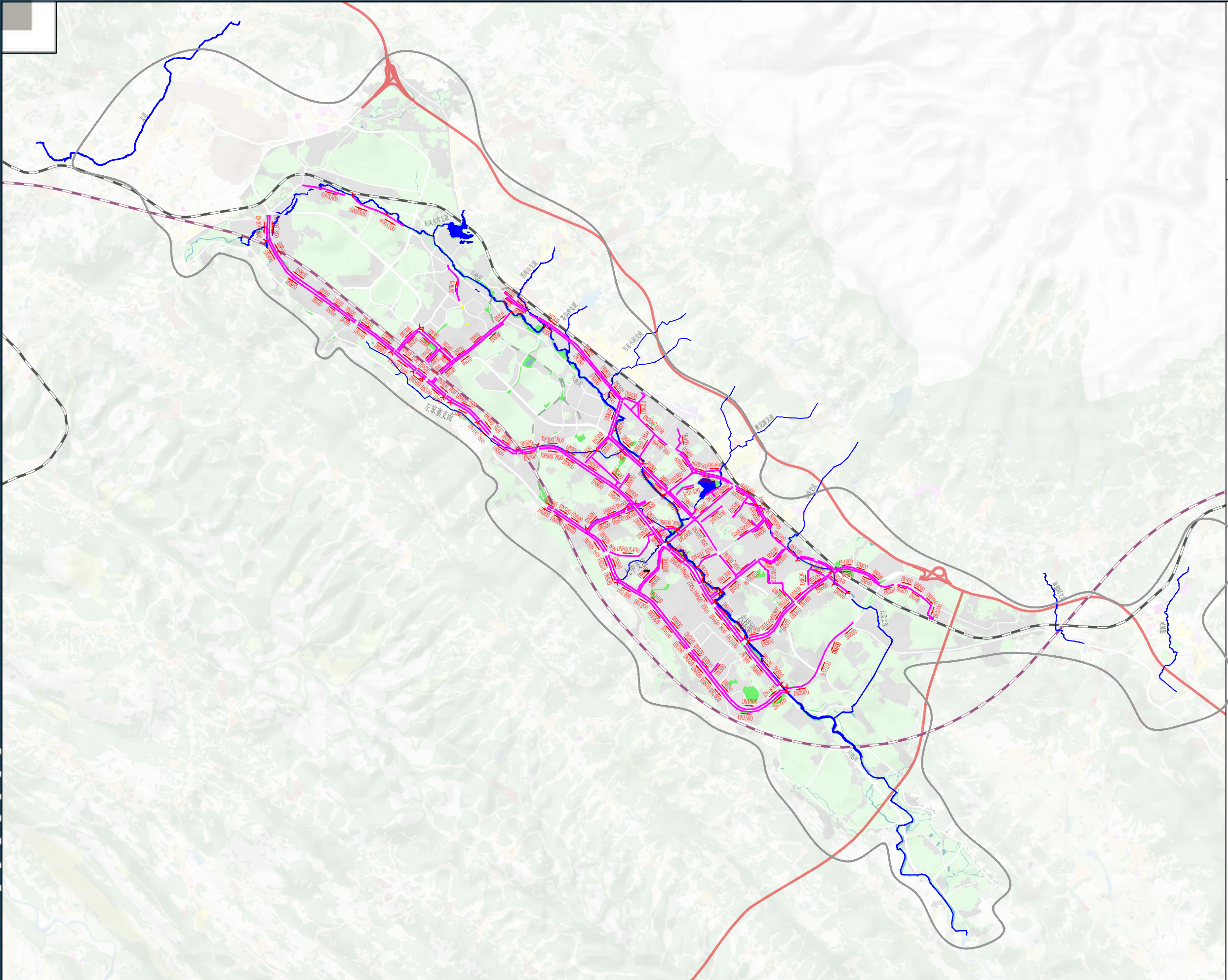
雨-02 中心城区雨水系统现状分布图
