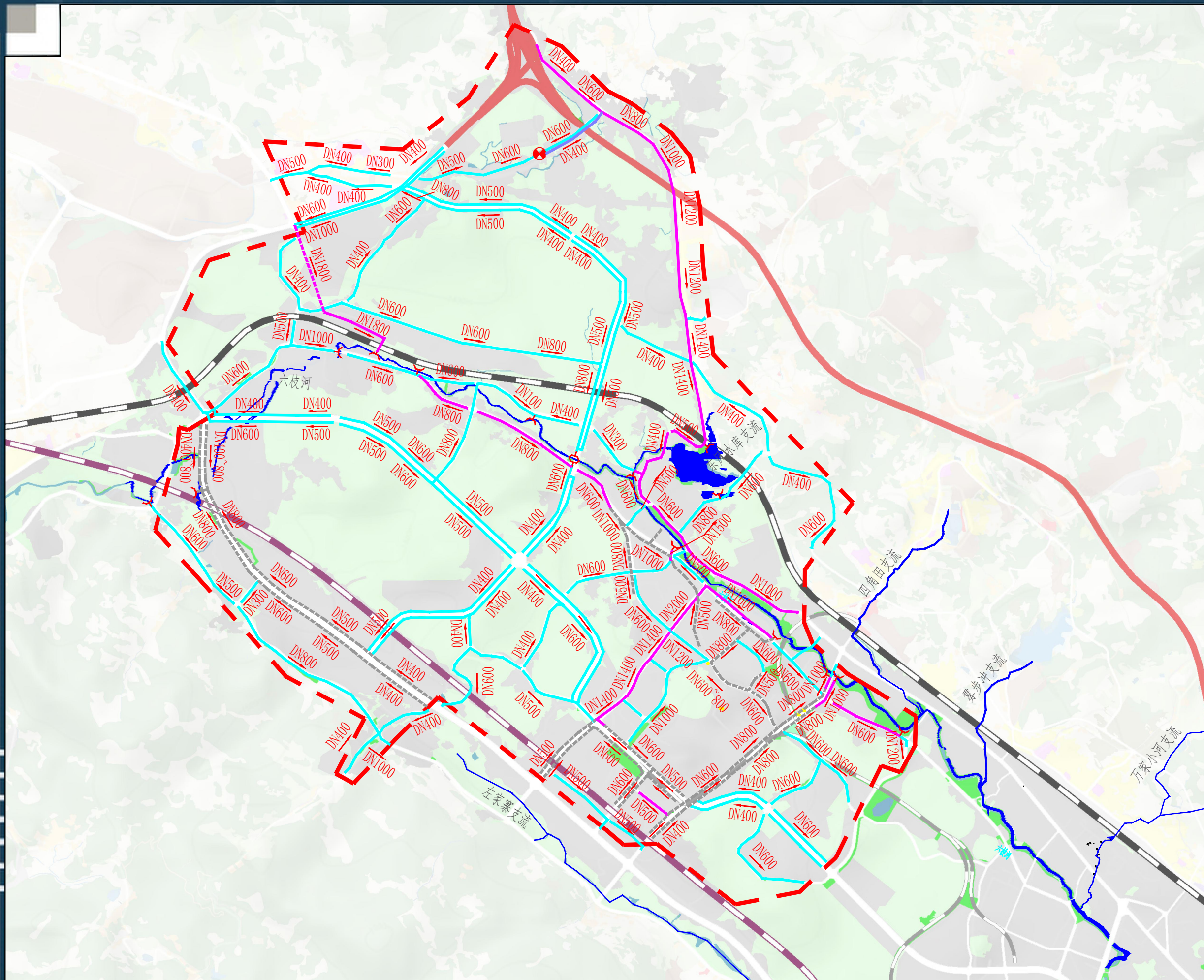
雨-04 十中-那玉片区雨水管网规划图
