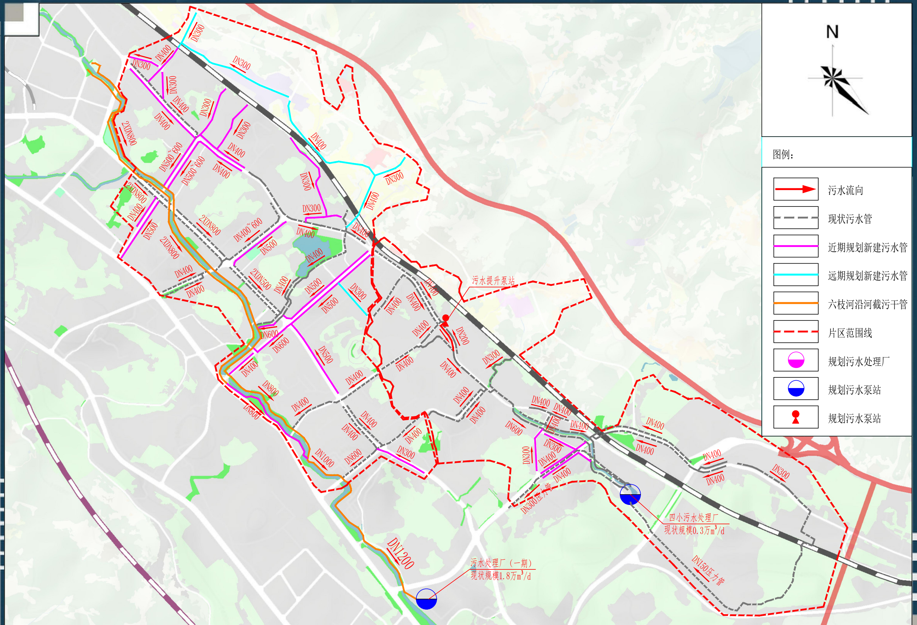
污-06 那平路、四小片区污水管网规划图
