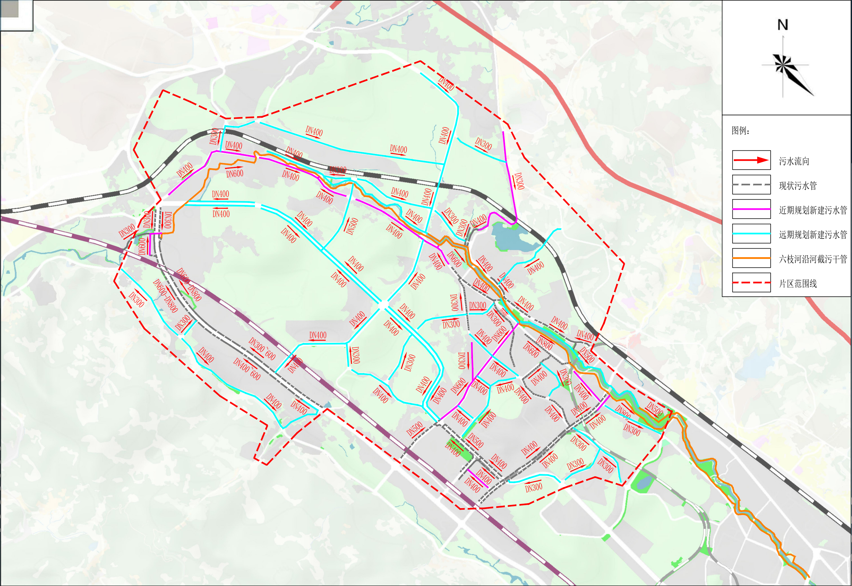
污-04 十中-那玉片区污水管网规划图
