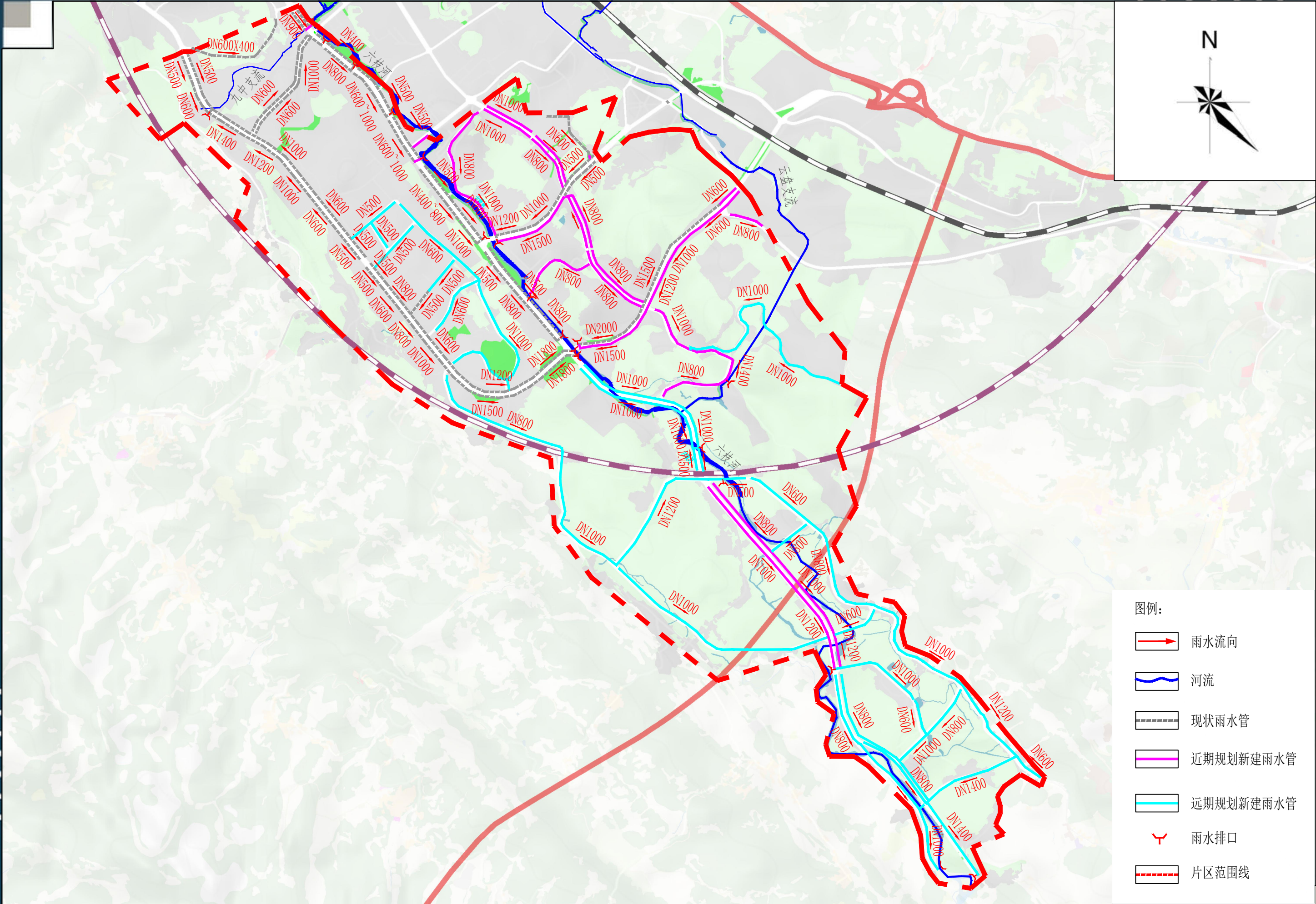
雨-08 牂牁大道东片区雨水管网规划图
