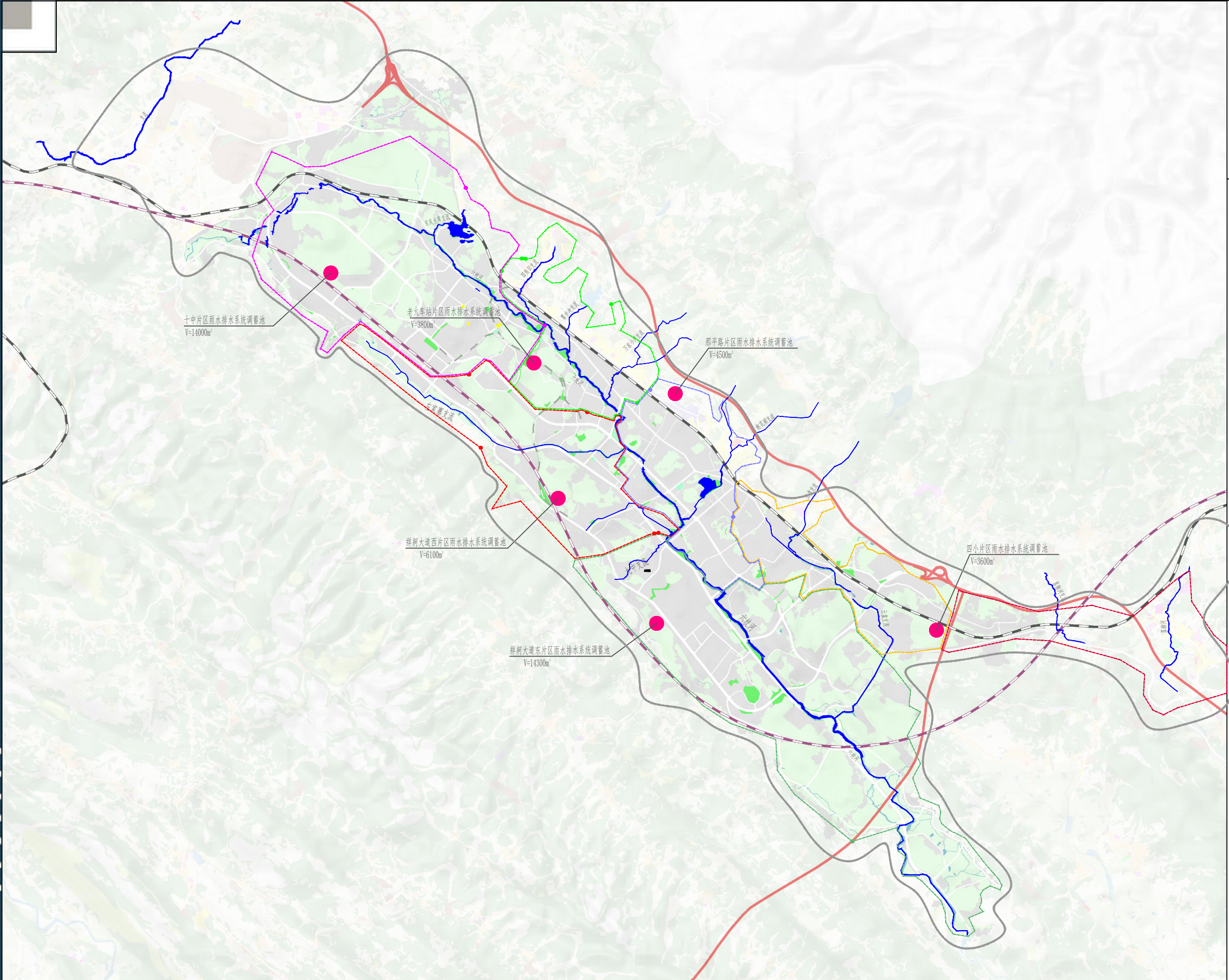
雨-11 中心城区雨水调蓄池规划分布图
