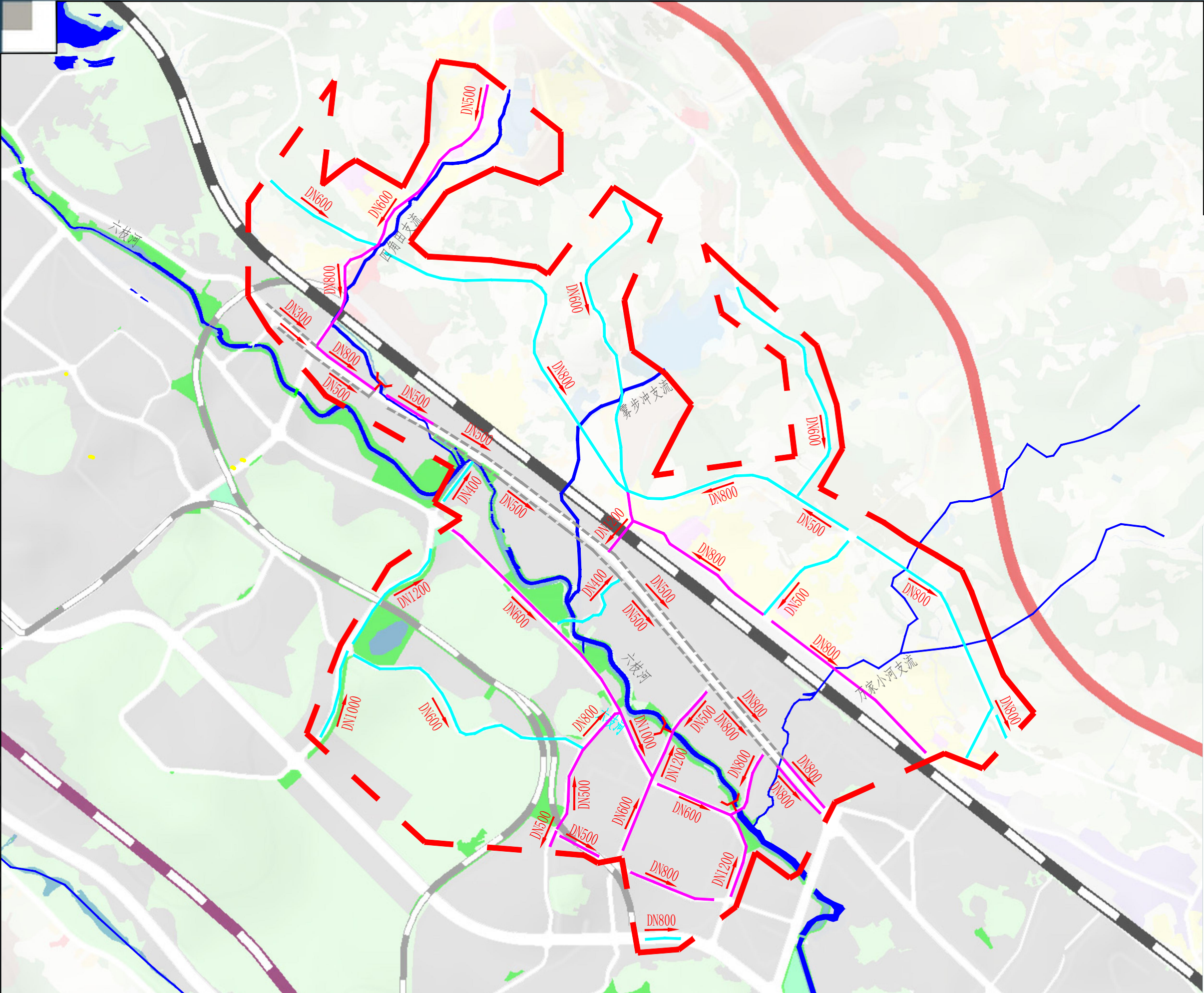
雨-05 老火车站片区雨水管网规划图
