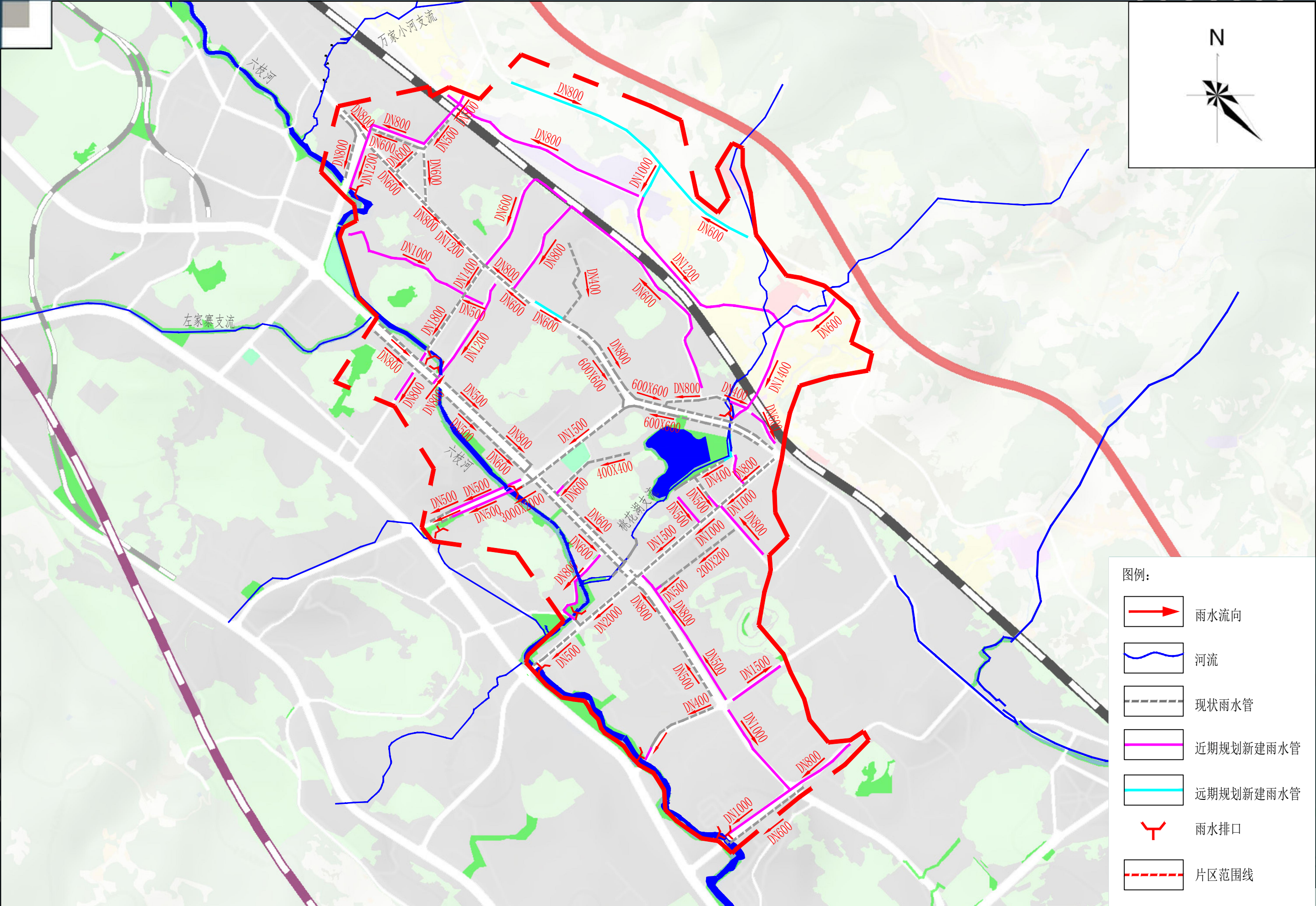
雨-06 那平路片区雨水管网规划图
